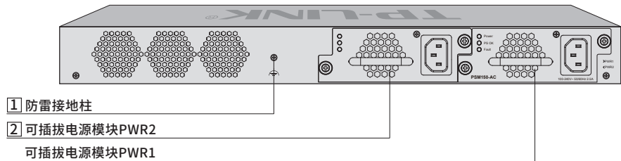
图1-11 TL-NS680-24T2Q后面板示意图
