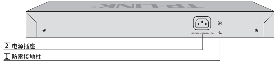
图1-15 后面板示意图
